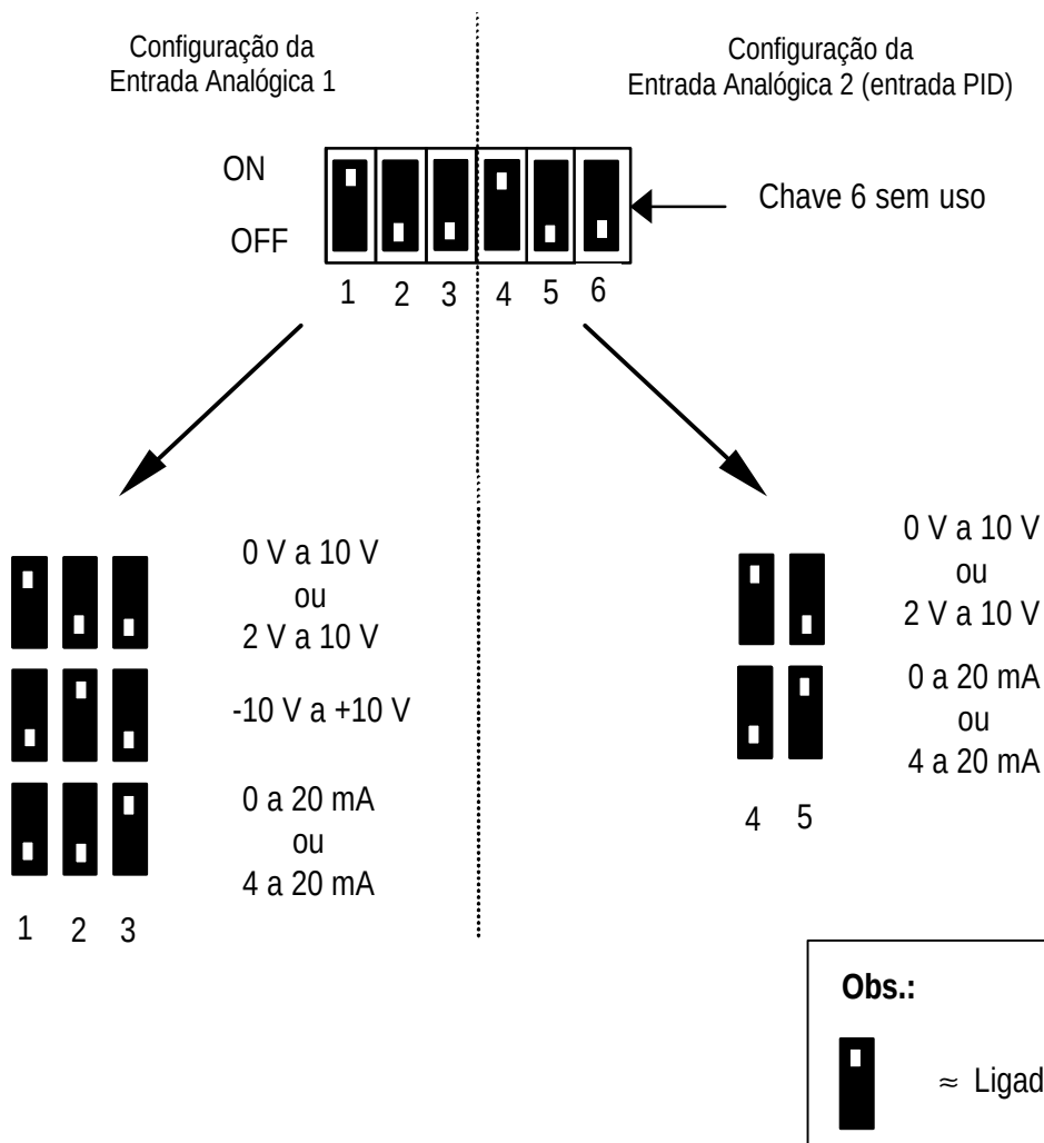
Figura 16. Microchaves Seletoras
