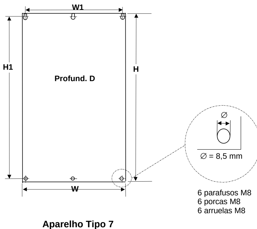
Figura 10: Dimensões para Montagem - MIDIMASTER Vector
